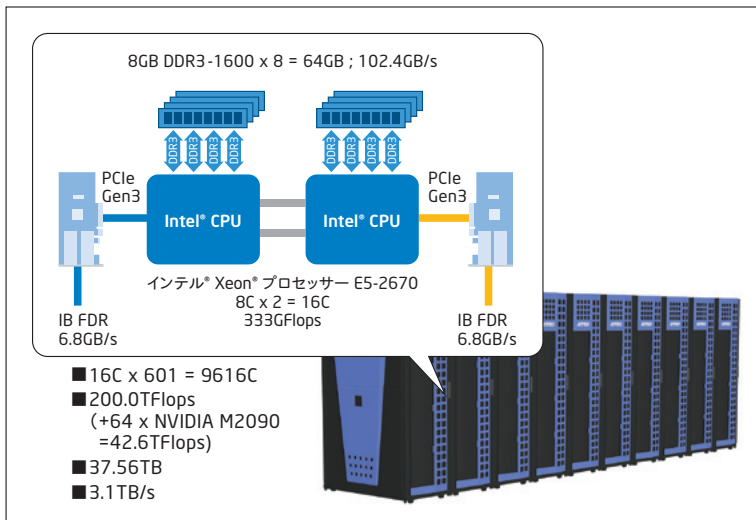
図 3. 601 台のノードで構成されたサブシステム Laurel の構成
