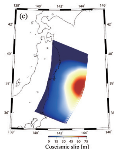
図 1. 巨大地震のシミュレーション計算画像
