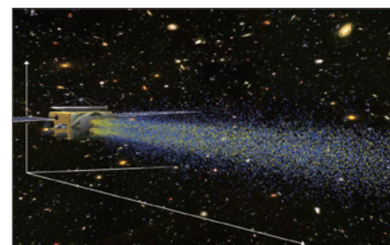
図 2. イオンエンジンとプラズマの相互作用に関する、大規模粒子シミュレーション
