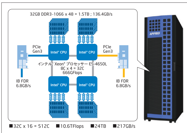
図 4. 1.5TB のメモリーを搭載した 16 台のノードで構成されたサブシステム Cinnamon の構成
